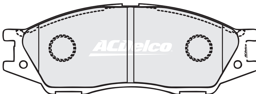
ACD1454 (15.1mm) NISSAN
